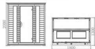
06-B61 Size: 1800×1300×2000mm
