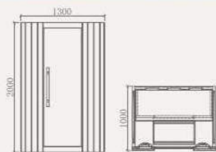
O2-K2 Size: 1300×1000×2000mm
