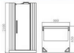
HW90 Size: 850×900×2100mm
