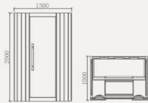
02-K2 Size: 1300×1000×2000mm
